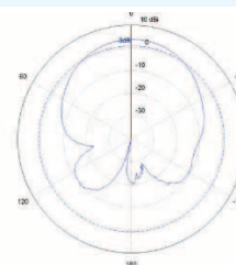
Antenne met circulaire polarisatie.
